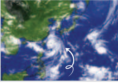
Tayfunun uydu görüntüsü
