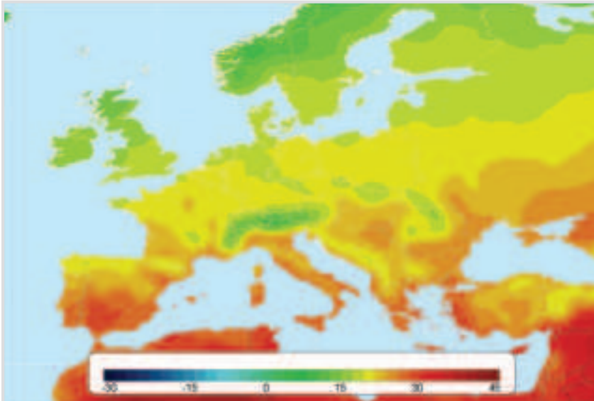
Avrupa’da Sıcaklıklar (°C)
